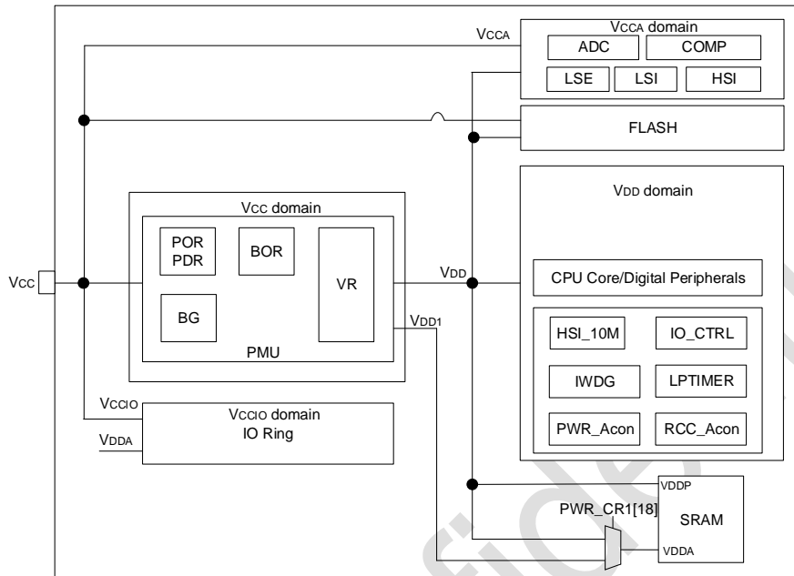
图 2-2 电源框图
