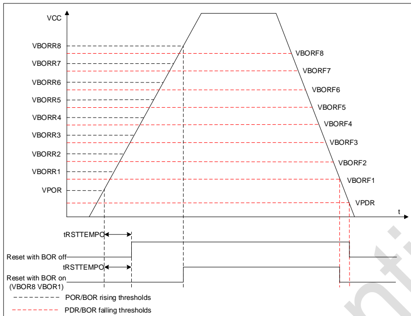
图 2-3 POR/PDR/BOR 阈值
