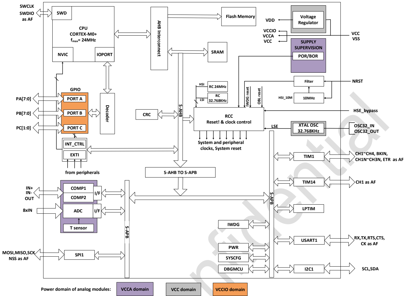
图 1-1 功能模块
