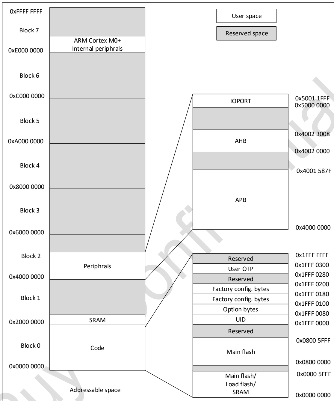
图 4-1 存储器映射
